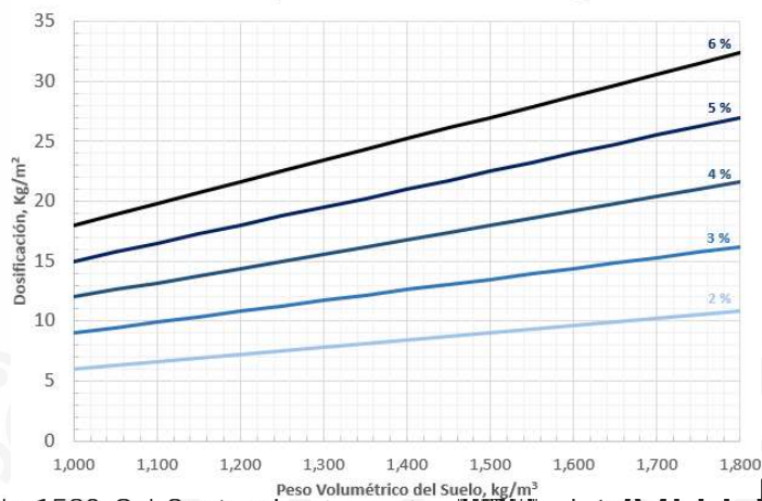
Dosificación por Relación de Cal @30cm
